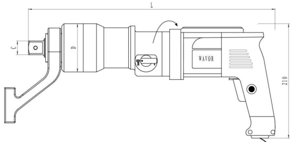
ETW直柄电动扳手尺寸示意图
